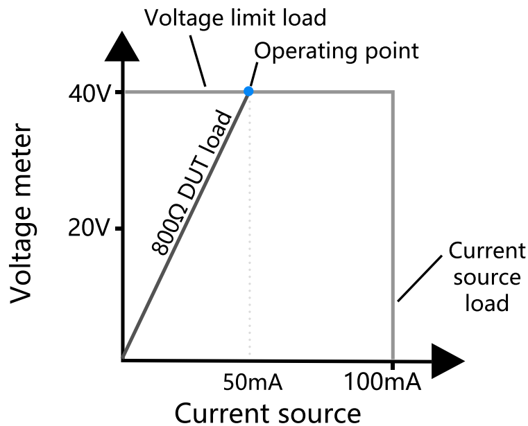
图 8. OE8101 电压限制边界示例
