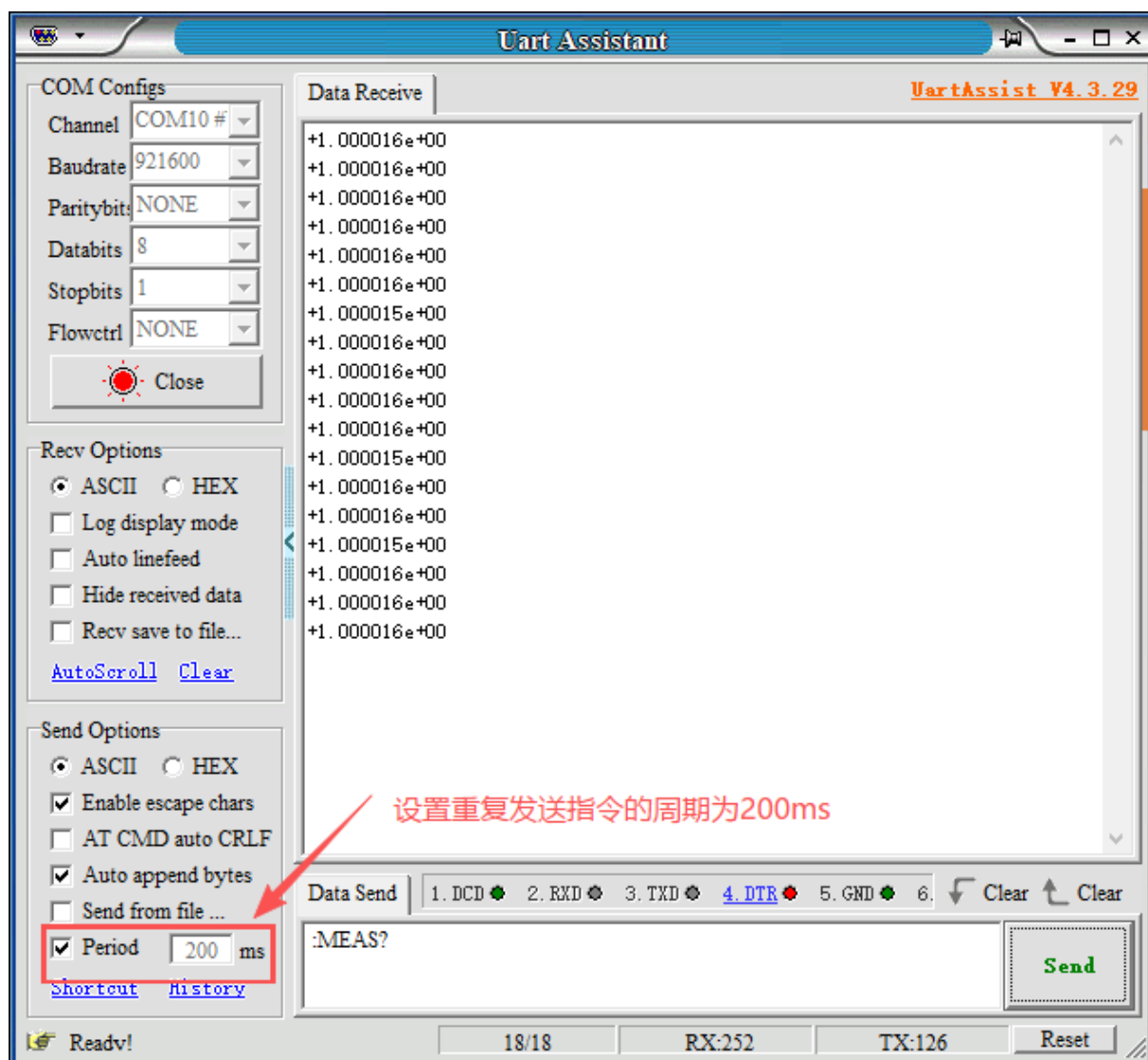
图 62. 连续读取测量值
