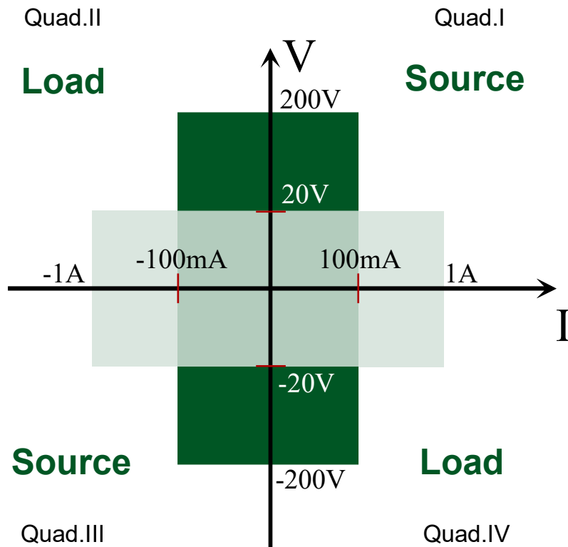
图 5. OE8101 功率包络
