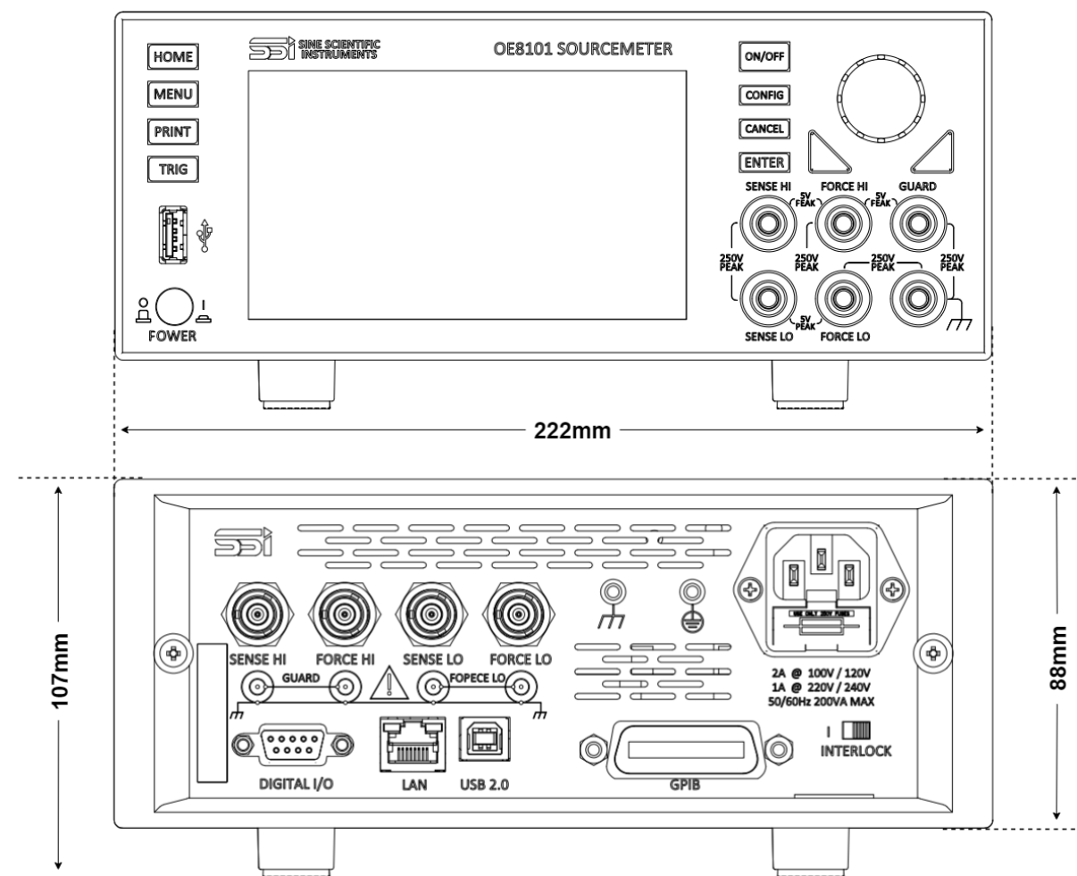
图 3. 前面板与后面板尺寸
