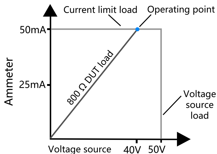
图 10. OE8101 电流限制边界示例
