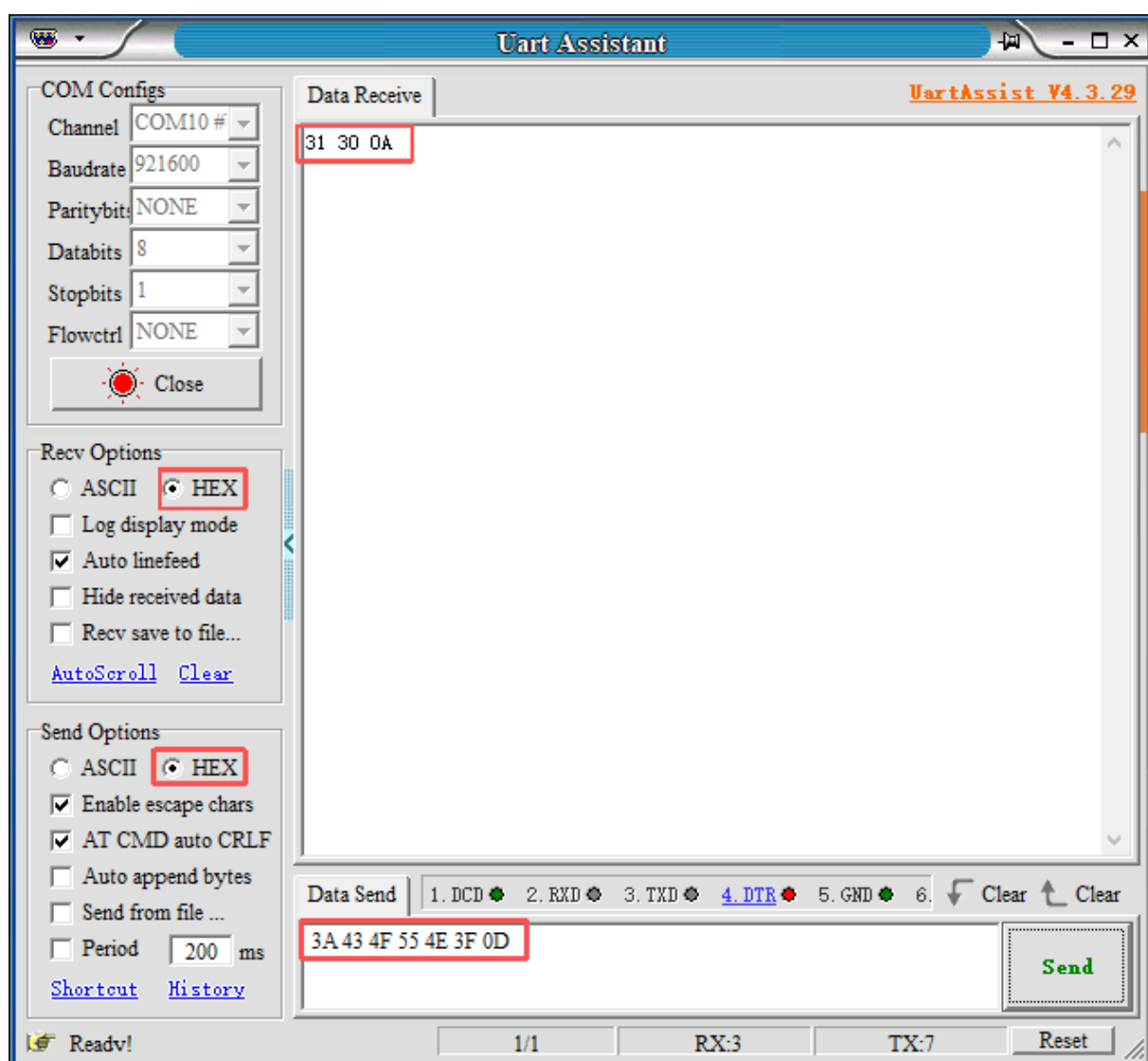
图 59. 十六进制格式发送指令和接收响应
