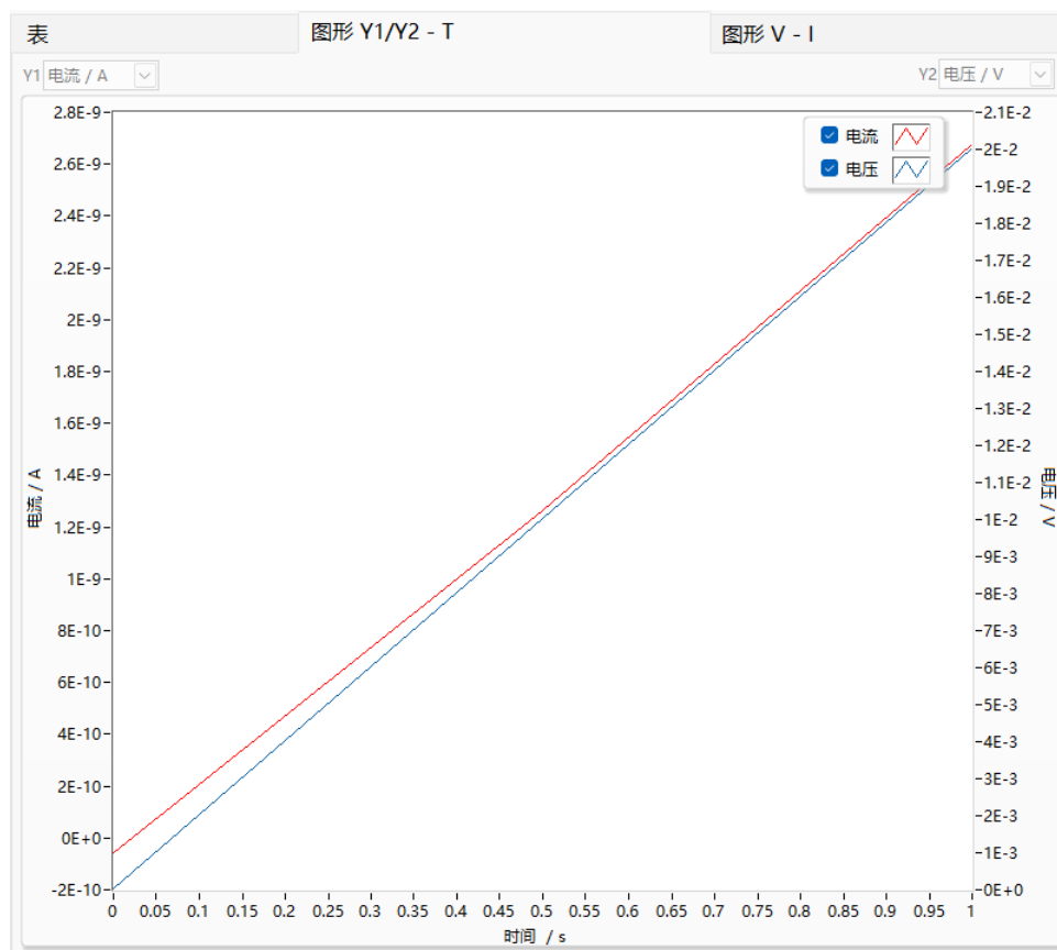
图 53. Y1/Y2-T 曲线
