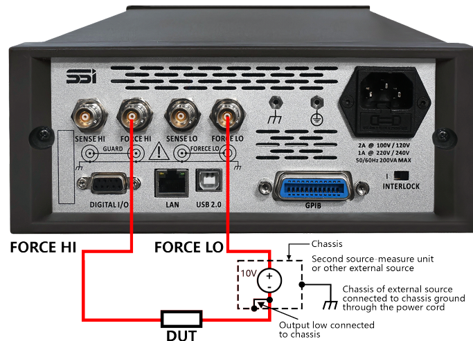
图 42. 仪器浮地示意图
