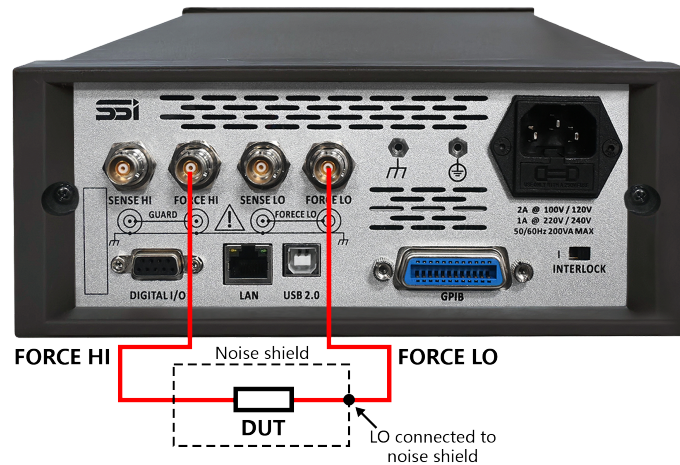
图 39. OE8101 后面板噪声屏蔽连接
