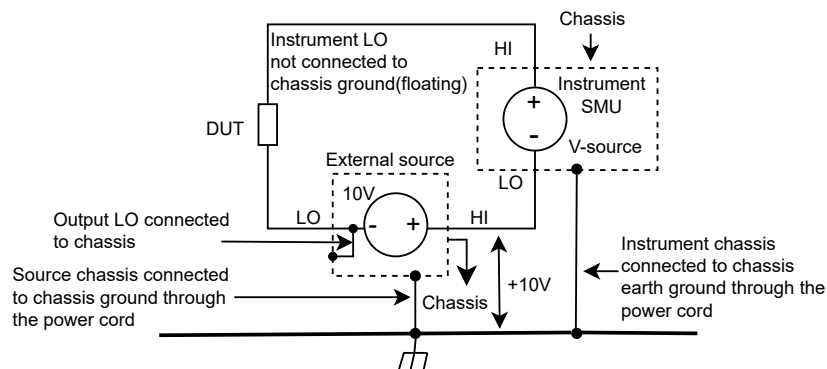
图 41. 仪器浮地示意图
