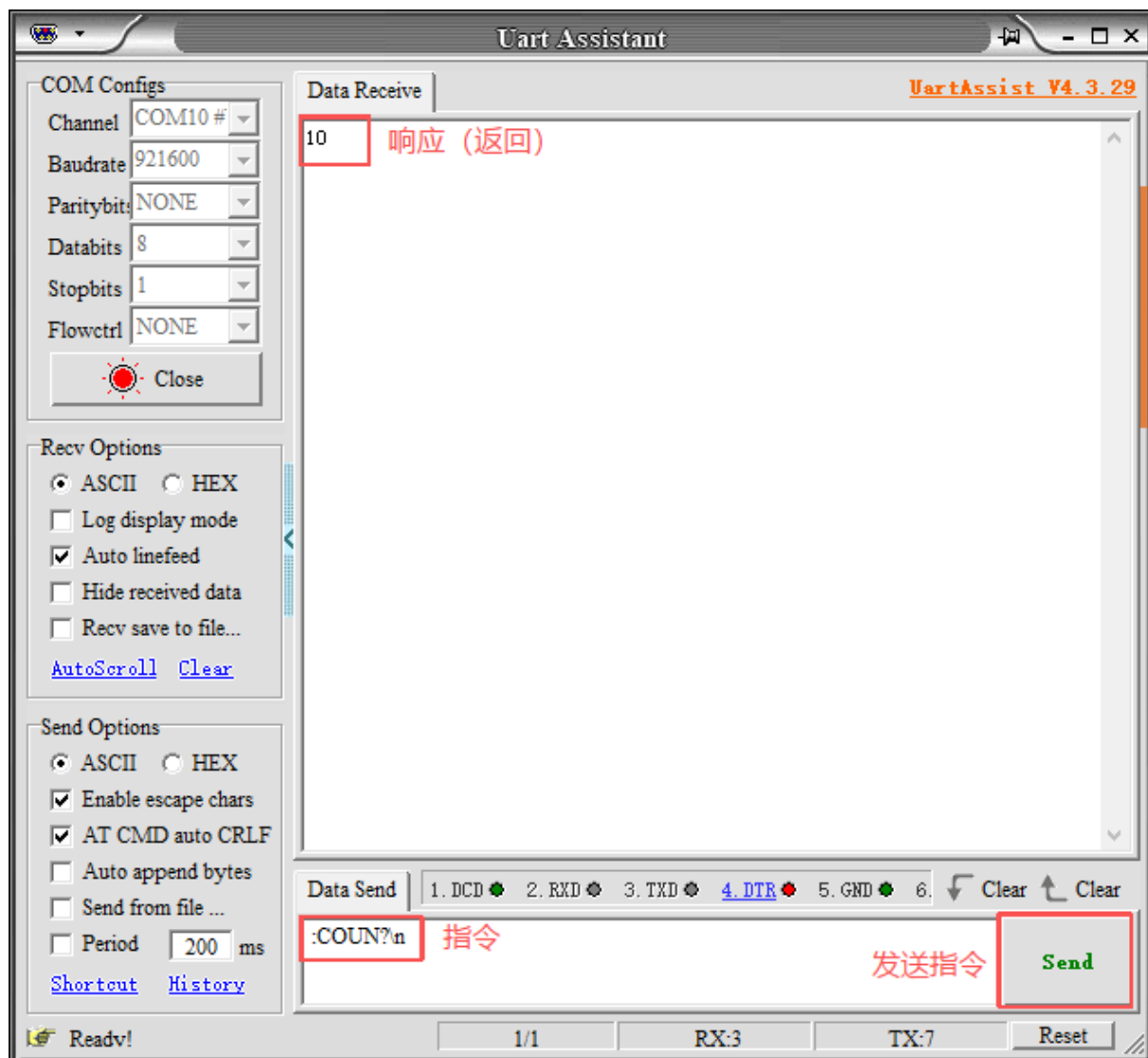
图 58. ASCII 码形式发送指令和接收响应
