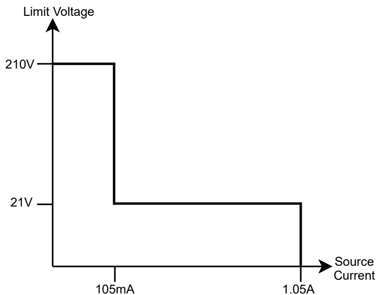
图 6. OE8101 电流源输出特性
