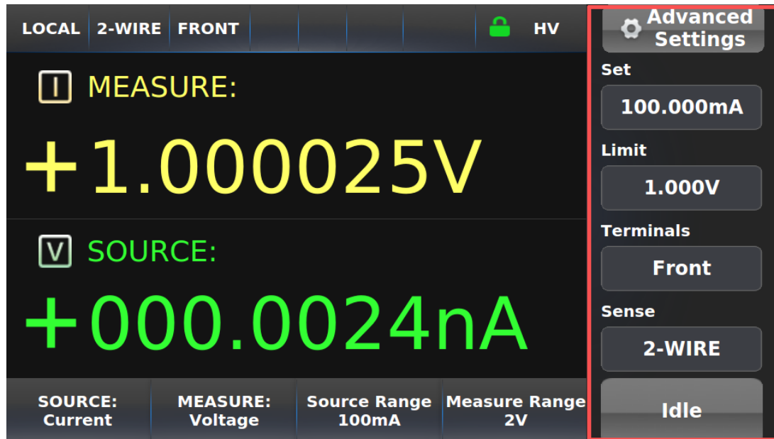
图 13. 主界面右侧功能设置区
