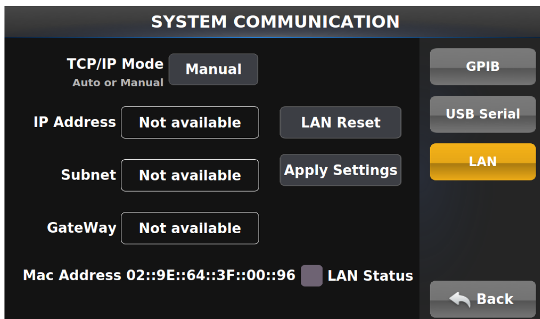
图 33. LAN 配置界面
