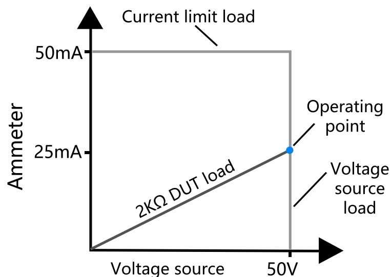
图 9. OE8101 电流限制边界示例-正常
