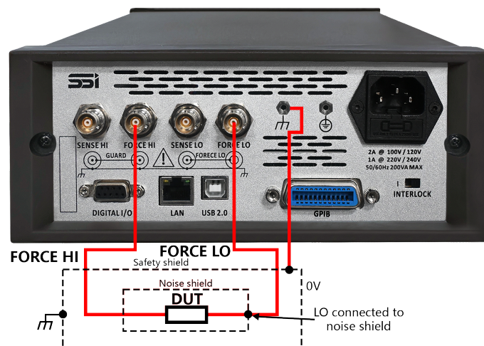
图 40. OE8101 噪声屏蔽和安全屏蔽
