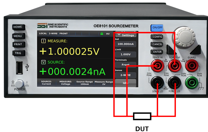
图 37. 前面板四线连接
