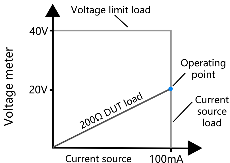
图 7. OE8101 电压限制边界示例
