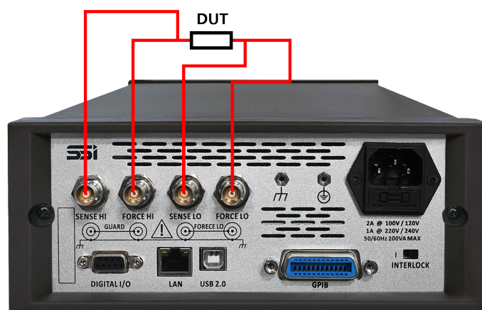
图 38. 后面板四线连接
